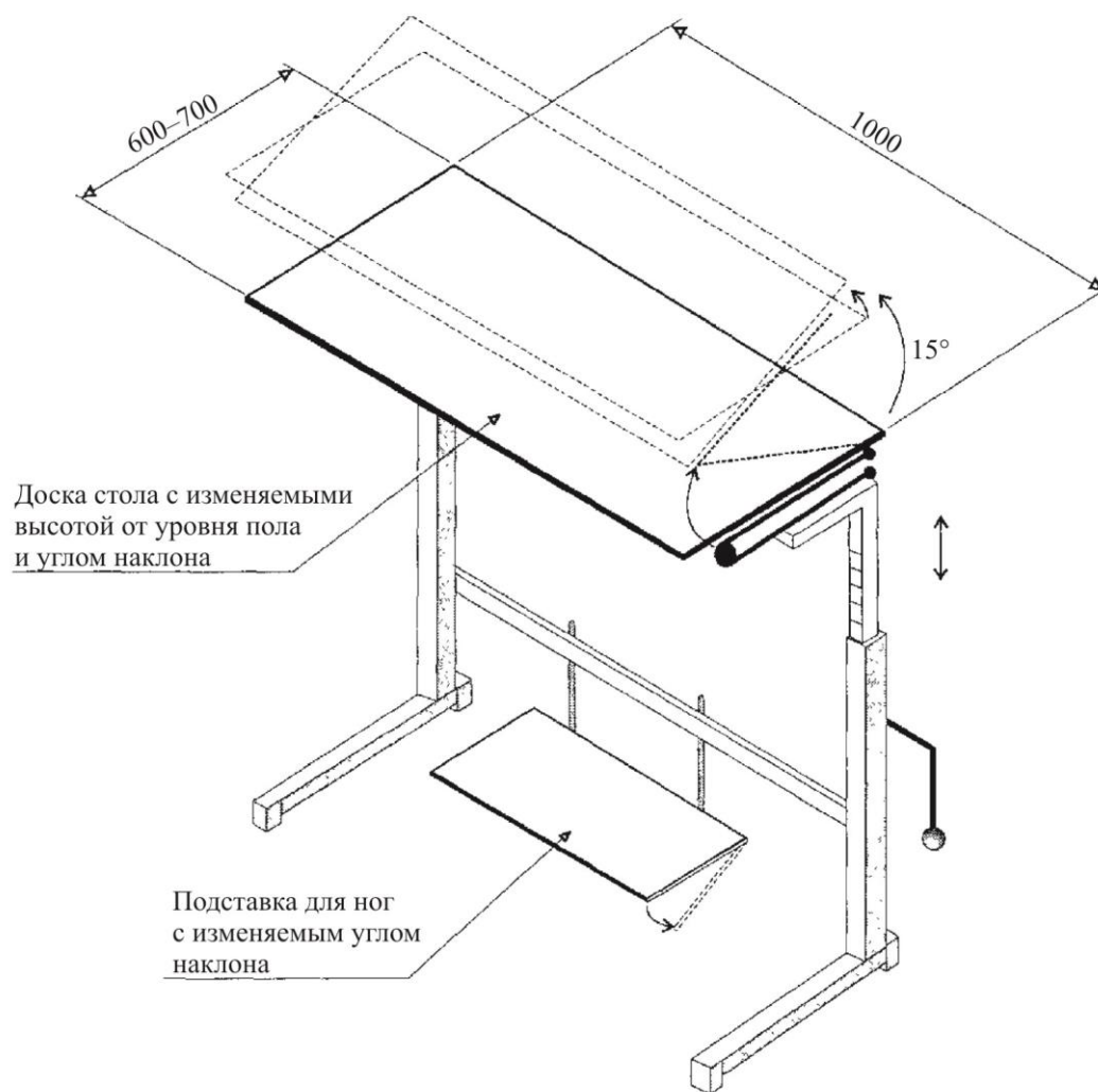
Рисунок В.12 – Трансформируемый рабочий стол для инвалида
